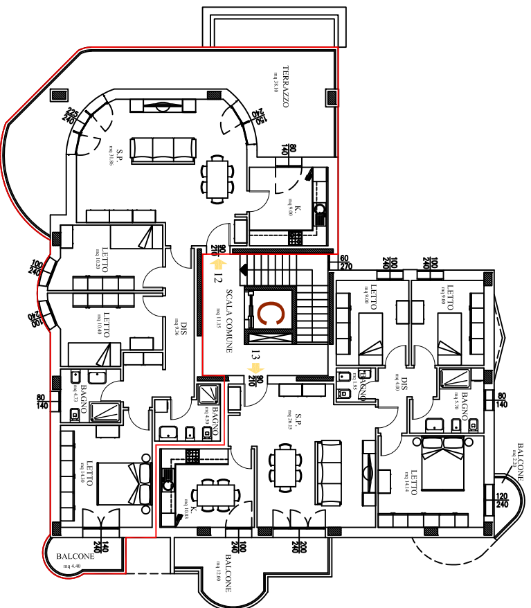
INQUADRAMENTO SCALA 1:200
