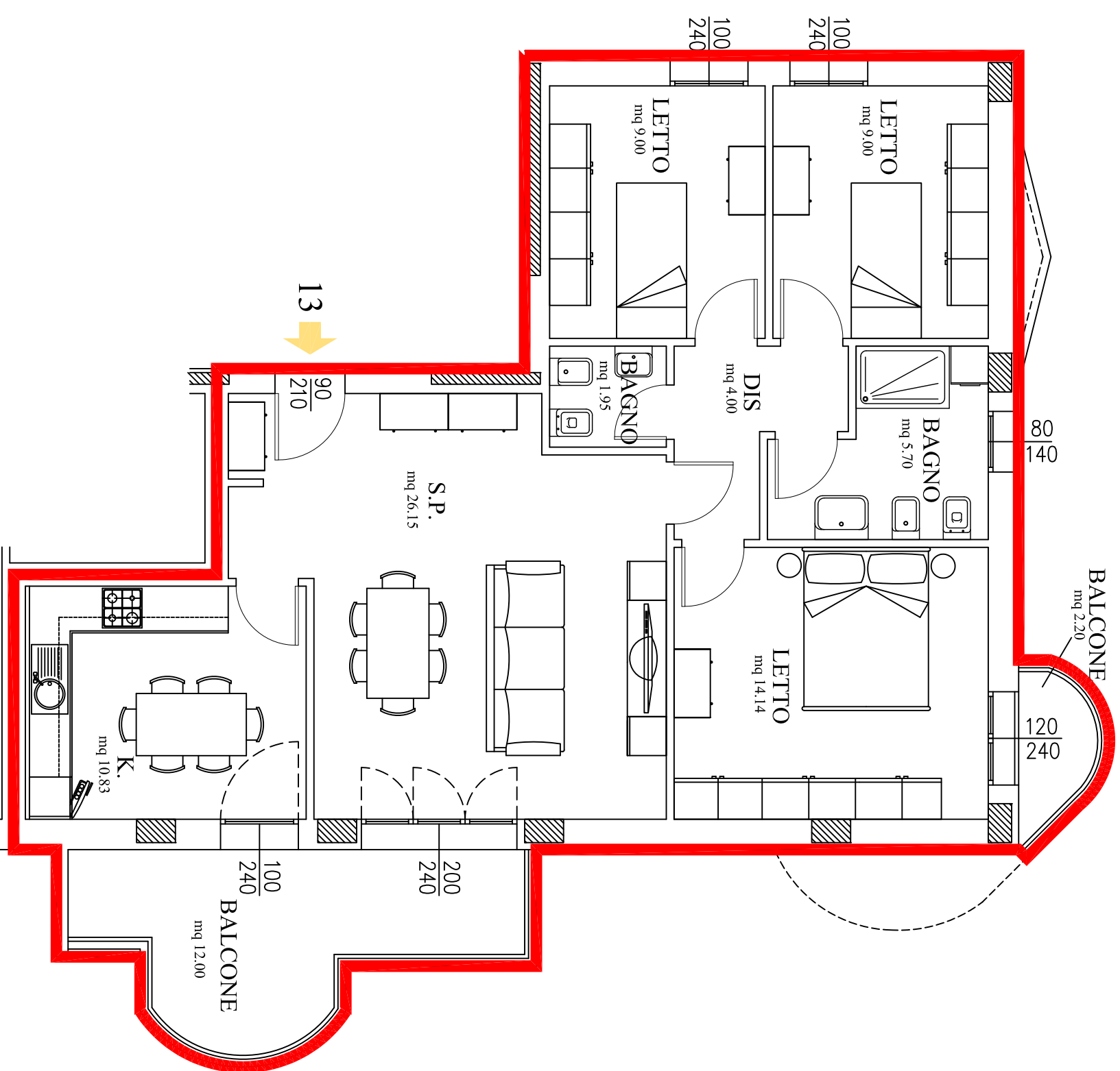
ALLOGGIO SCALA 1:66
