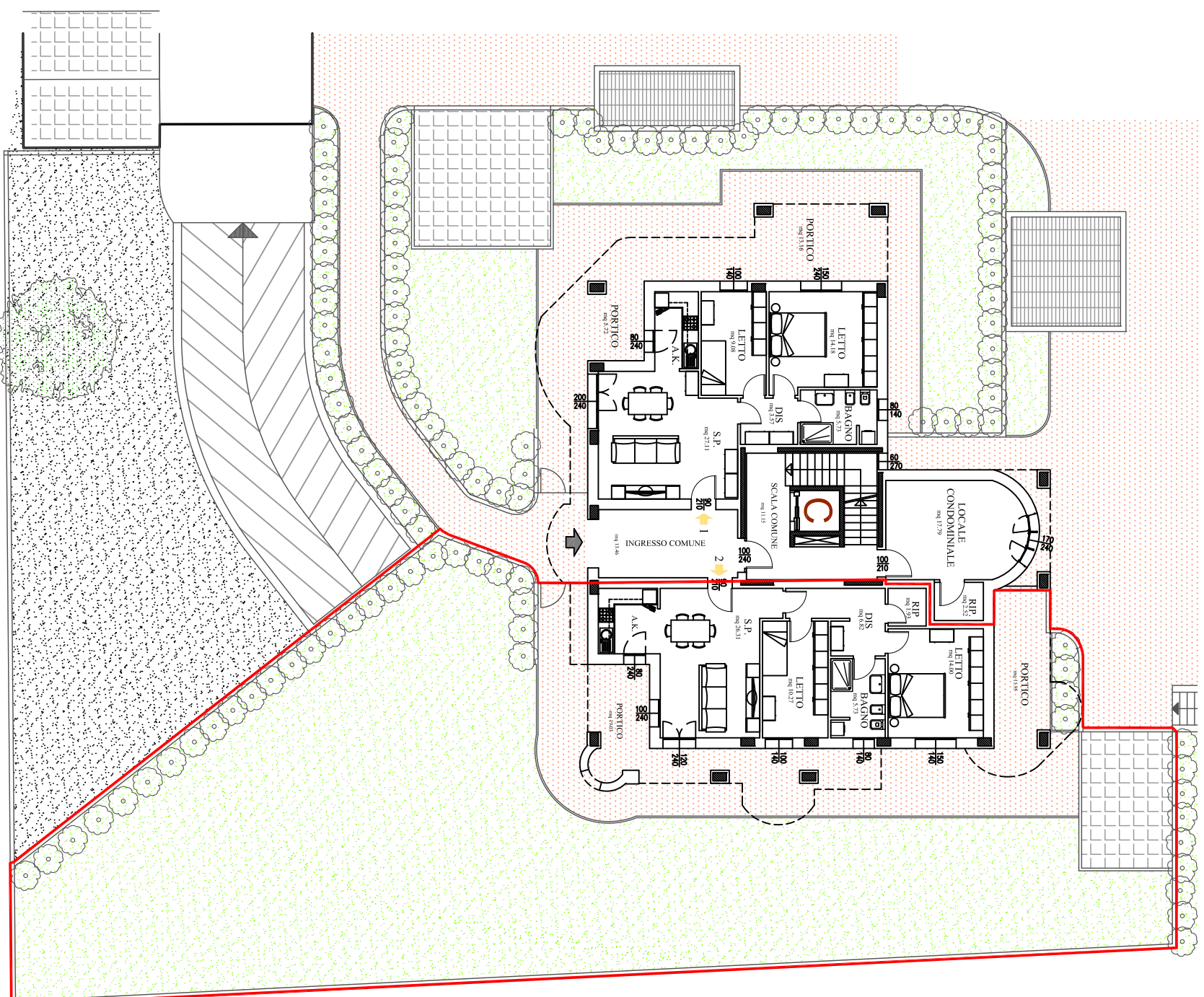
INQUADRAMENTO SCALA 1:200
