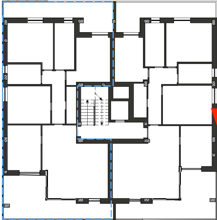
INQUADRAMENTO PIANO SECONDO Scala 1:200
