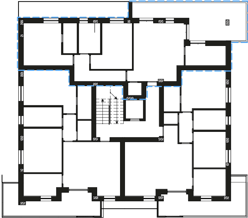
INQUADRAMENTO PIANO PRIMO Scala 1:200
