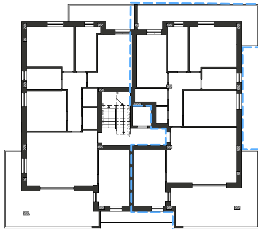
INQUADRAMENTO PIANO TERZO Scala 1:200
